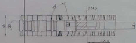
SEÇÃO 1-1
