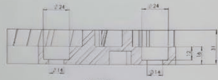
SEÇÃO a-a
