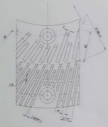
DETALHE c
